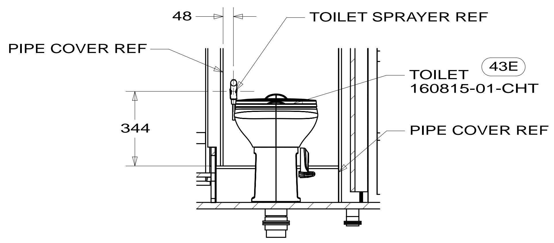
SECTION DC-DC
