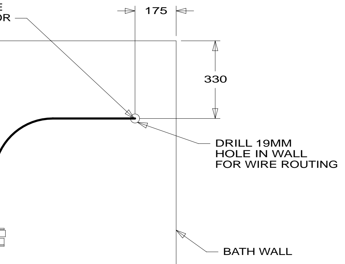
DETAIL AB 644
