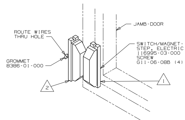
DETAIL EN
