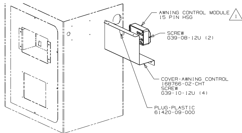
VIEW HA 52N
