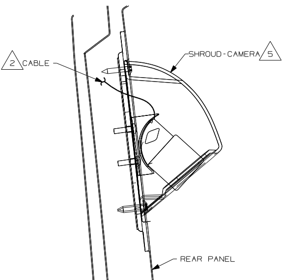
VIEW A-A
