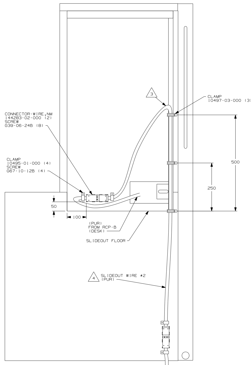
DETAIL DA
