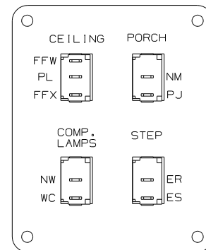
DETAIL DE
