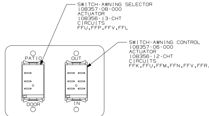
DETAIL DD
