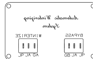
DETAIL DH
