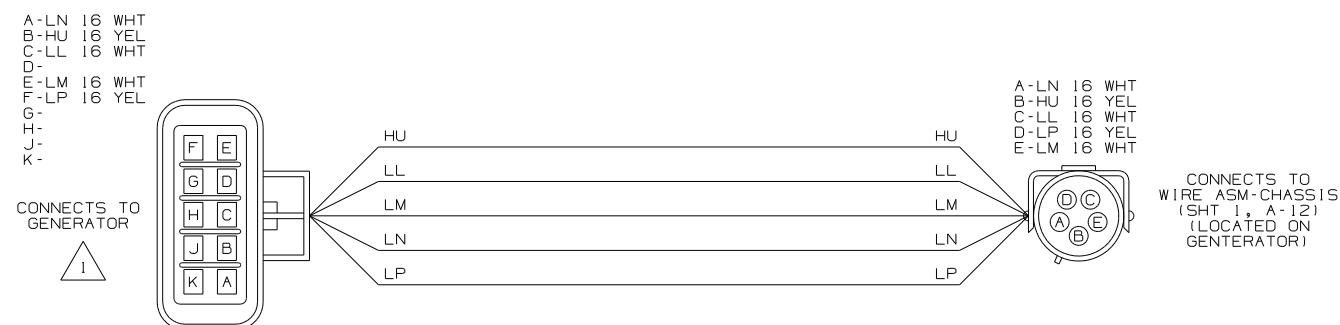
WIRING DIAGRAM-GEN ADAPTER,DIESEL WIRE ASM 130332-02
