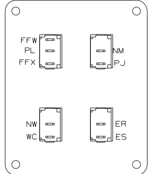
DETAIL EM (BACK SIDE)
