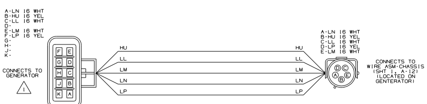
WIRING DIAGRAM-GEN ADAPTER,DIESEL WIRE ASM 130332-02
