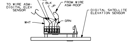
DETAIL GB (480)
