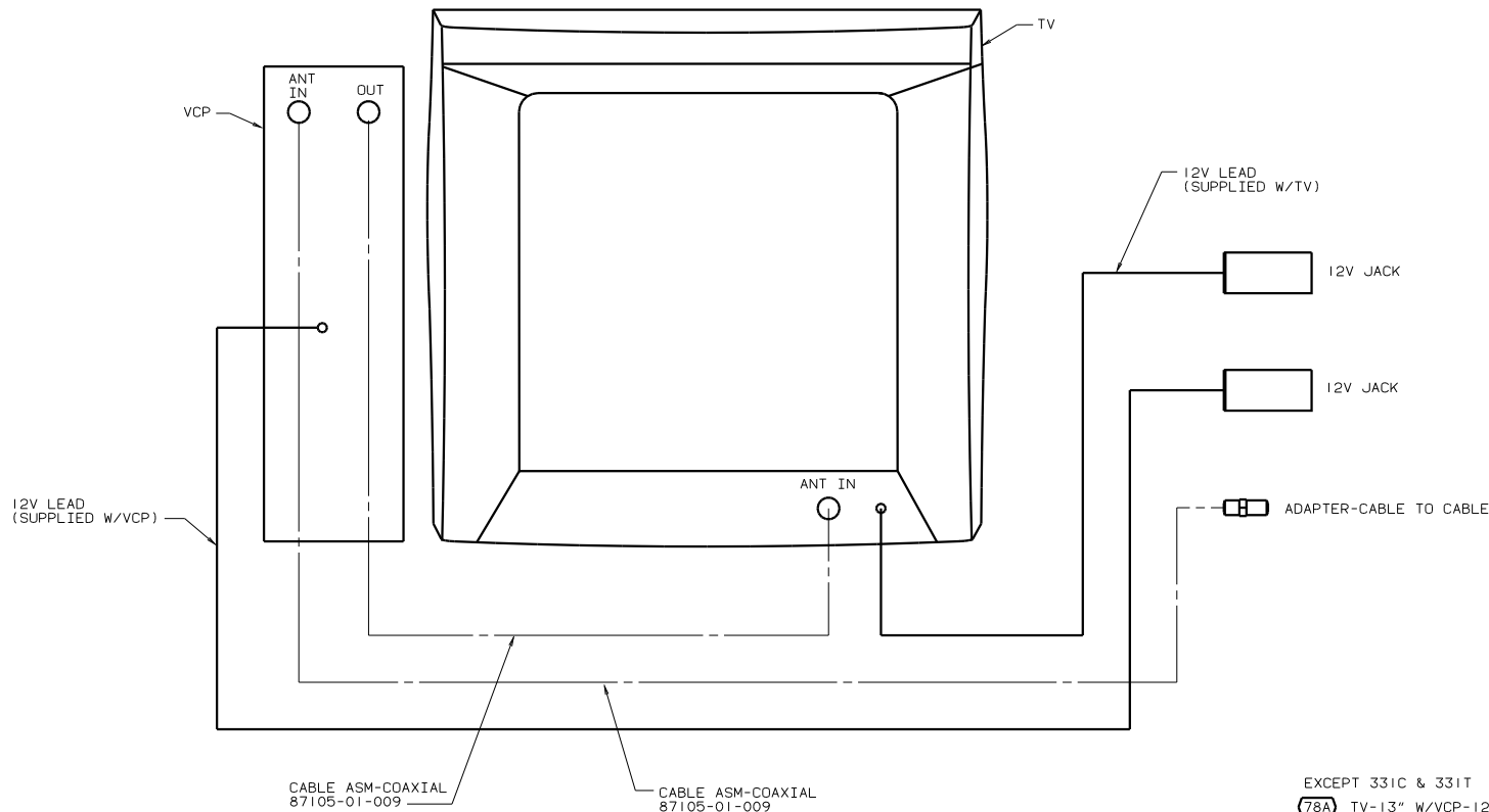
VIEW A-A
