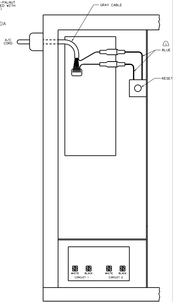
DETAIL DA-DA
