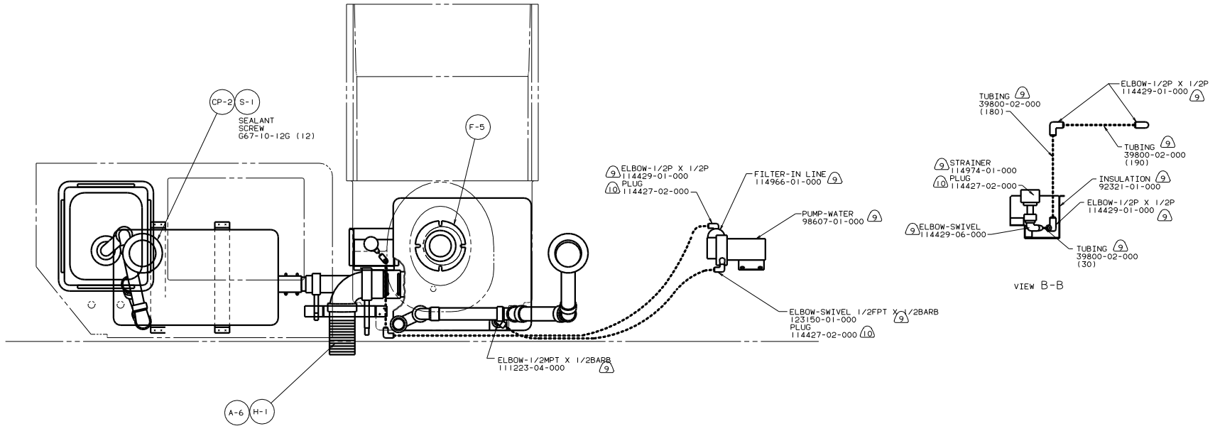
VIEW A-A
