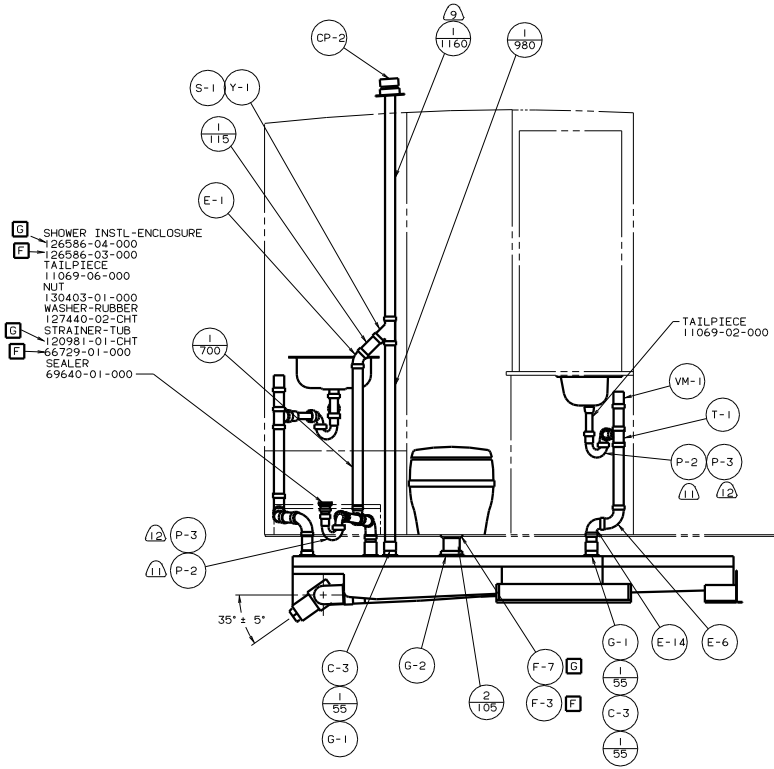
VIEW A-A
