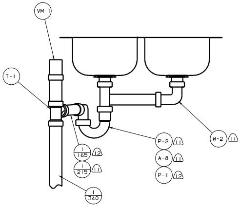
VIEW A-A
