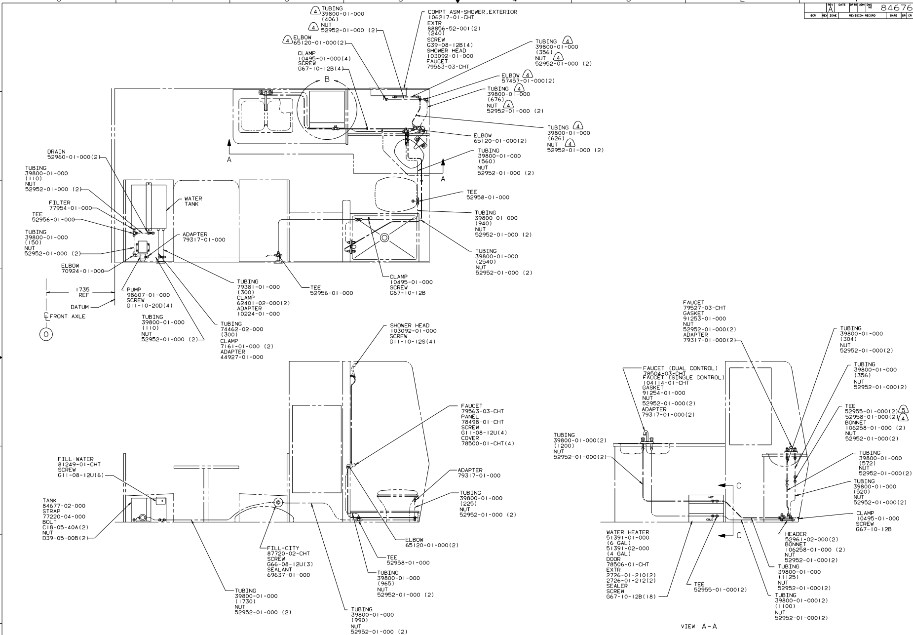
VIEW A-A
