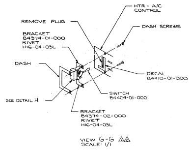
VIEW G-G SCALE: 1/1
