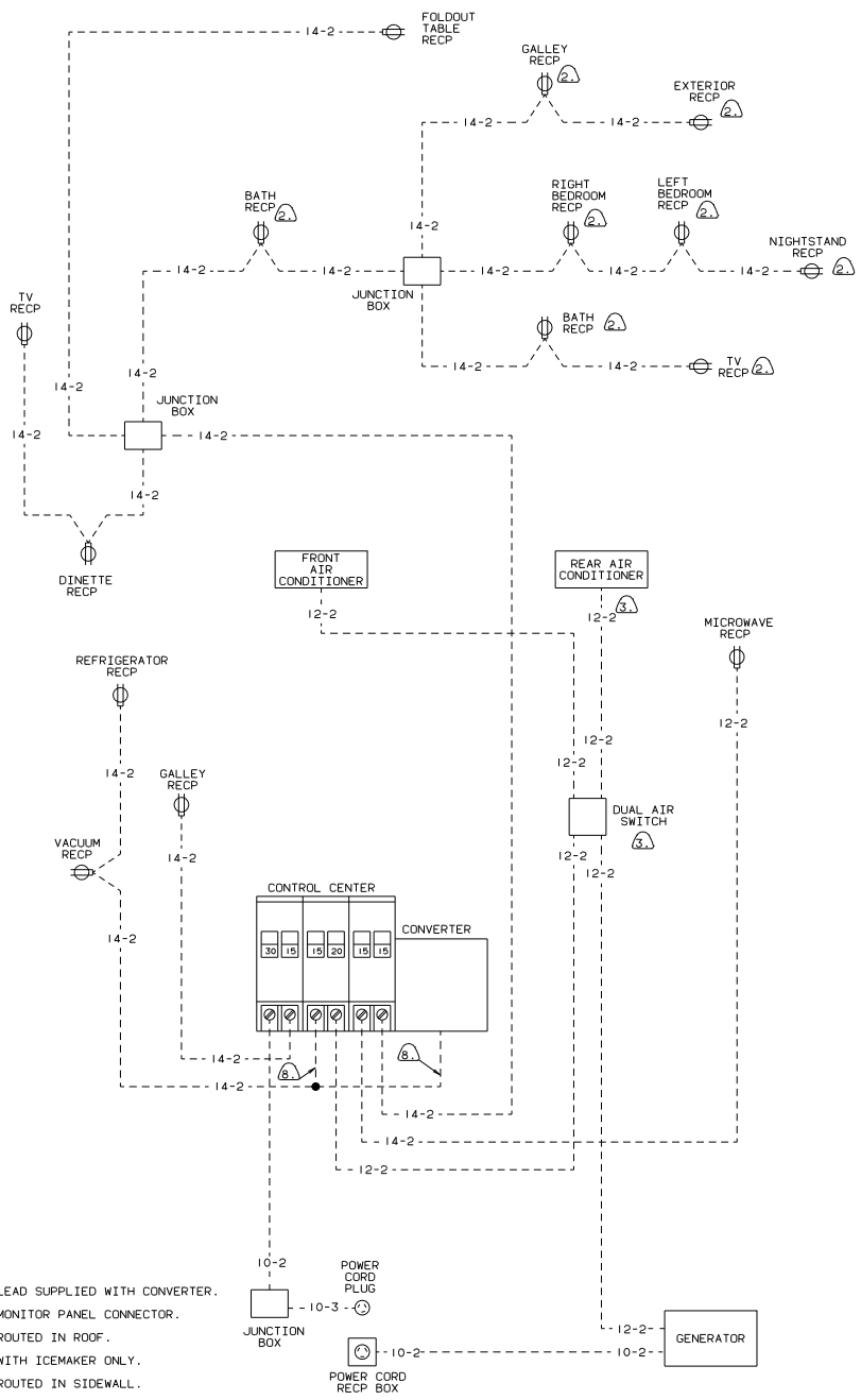
CAN 110 VOLT WIRING
