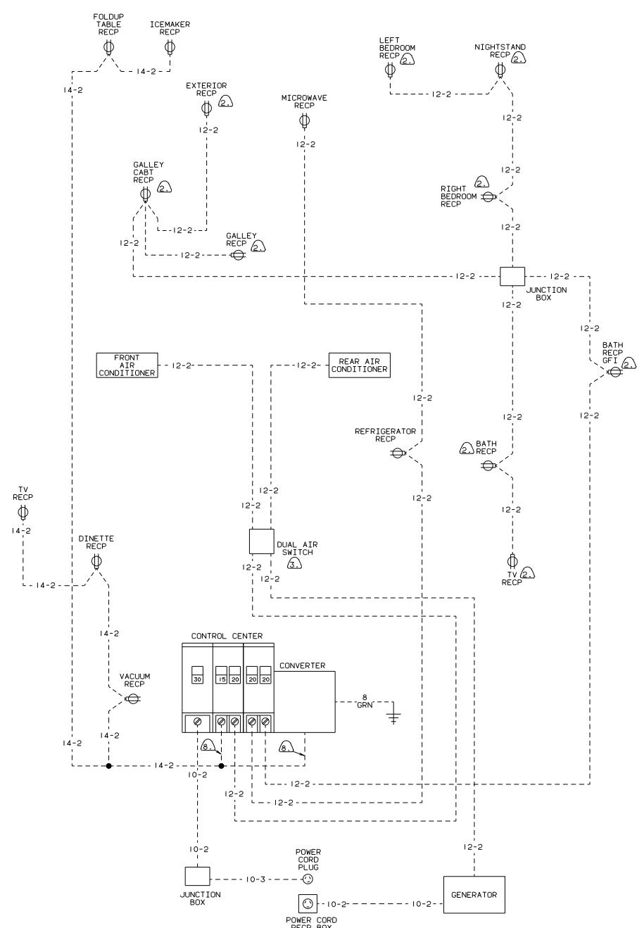
US 110 VOLT WIRING TWIN BED
