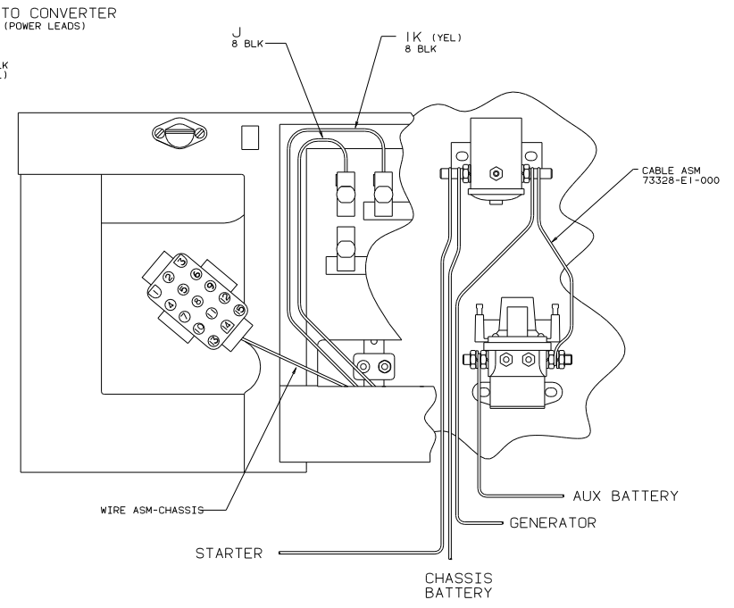
SECTION B-B SCALE: .8
